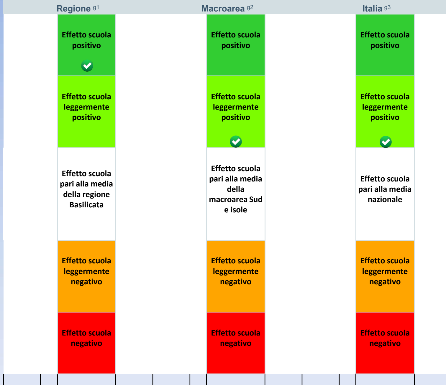
Grafico 6a: MTIC82000G - Scuola Secondaria di Primo Grado - Classi terze - Istituto nel suo complesso - Prova di Italiano - Effetto scuola calcolato rispetto a quello medio dei diversi aggregati territoriali di appartenenza
